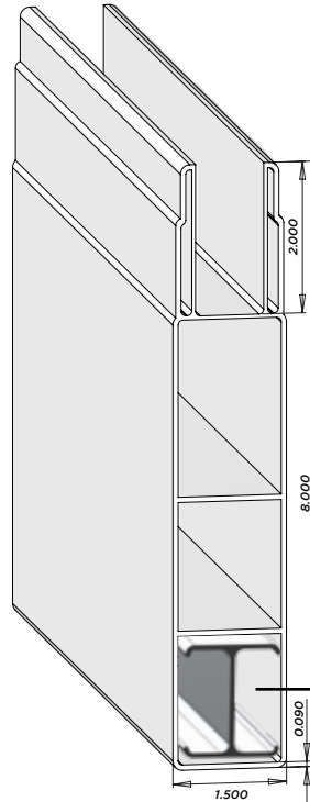
F3P1 1-1/2" x8" Gorilla® Pocket Rail 7/8" x 2" Deep Pcs/Pallet: 72 AL - NA NJ - NA UT - 76", 83", 88", 94", 16'
