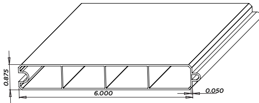
F54U (0.050 wall) 7/8"x6" T&G Utility Pcs/Pallet: 178 (16'), Shorter Lengths, 346 AL - 48", 52", 60", 61", 62-1/4", 64", 16' NJ - 48", 52", 60", 61", 62-1/4", 64", 16' UT - 48", 60-1/4", 62-1/4", 16'
