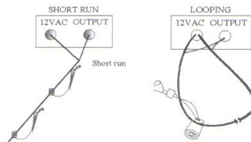
SCHÉMA 3B
