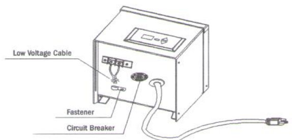
SCHÉMA 3
